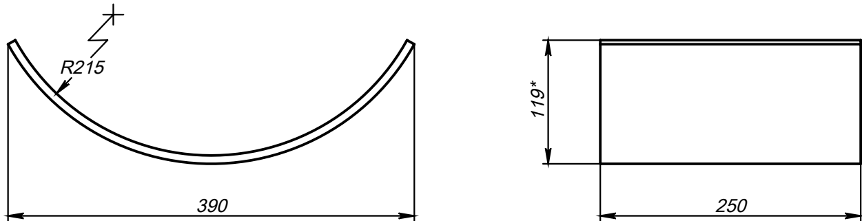
Поз.3 (Ложмент)
